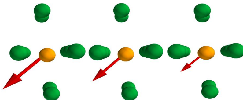
Figure II.4.8 : Représentation de l'évolution du vecteur DM dans les fragments CuCl 2 étudié en partant d'une déformation 0.15Å, 0.1Å à 0.06Å de gauche vers la droite.
